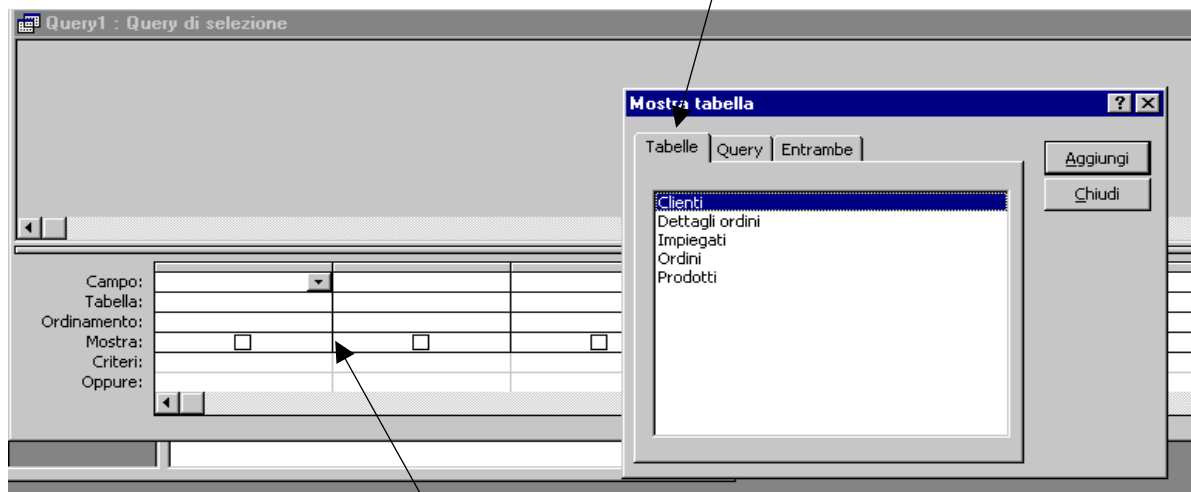
Griglia QBE
